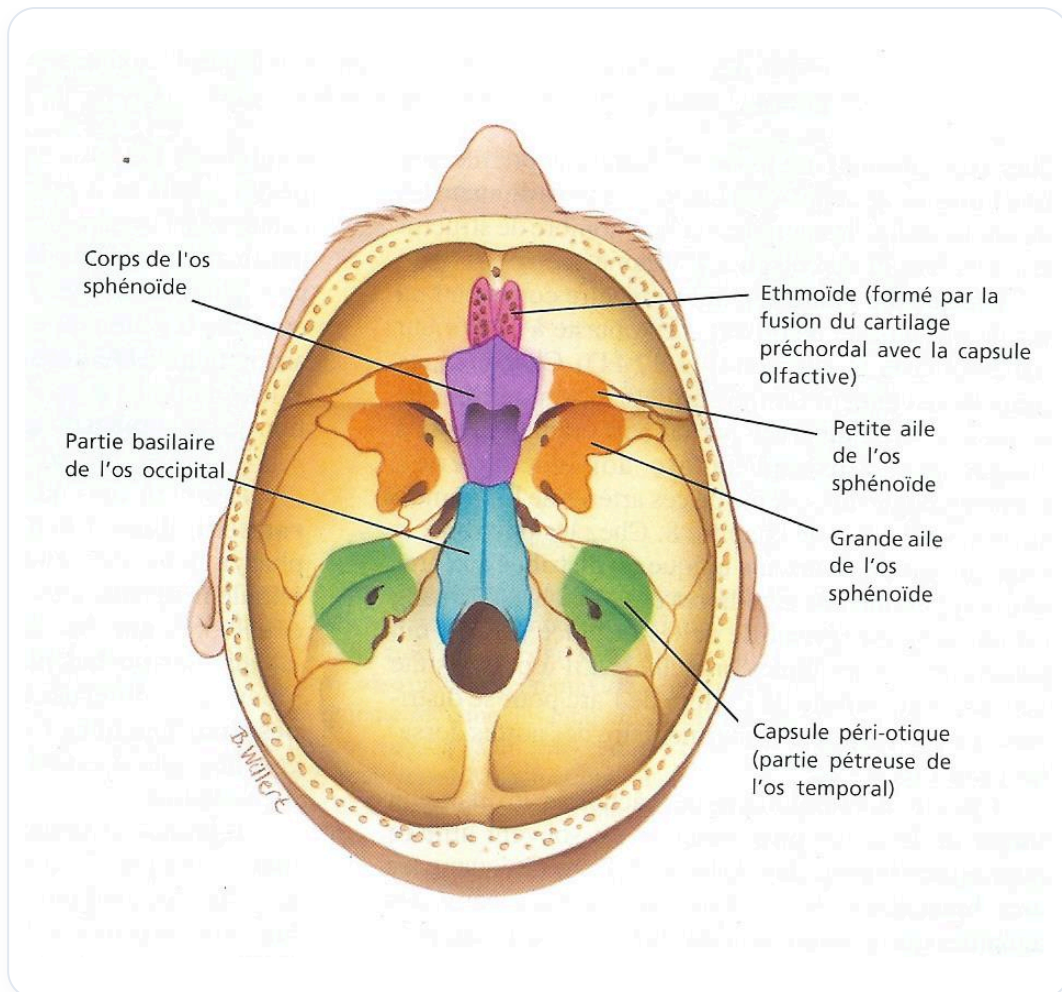
FIG. — Base cranica vista superiore
